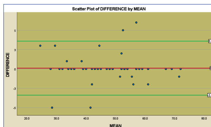
[Table/Fig-6]: Bland Altman Plot.
